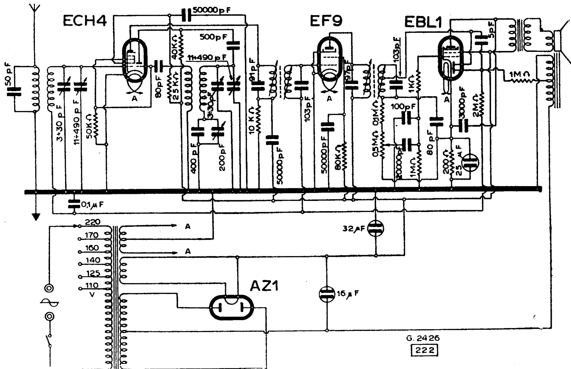
PHILIPS RADIO - MOD. « 333 »
